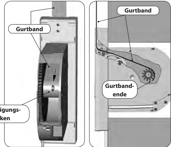
Gurtbandverlauf im RolloTron Standard
